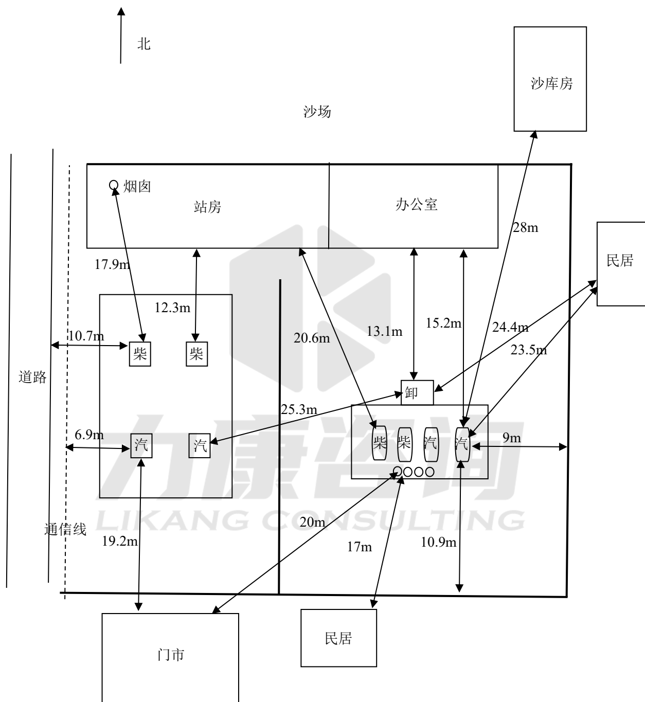
图 2.3-1 周边环境及总平面示意图
