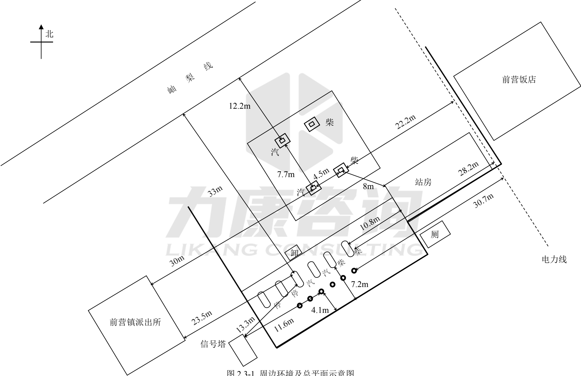
图 2.3-1 周边环境及总平面示意图
