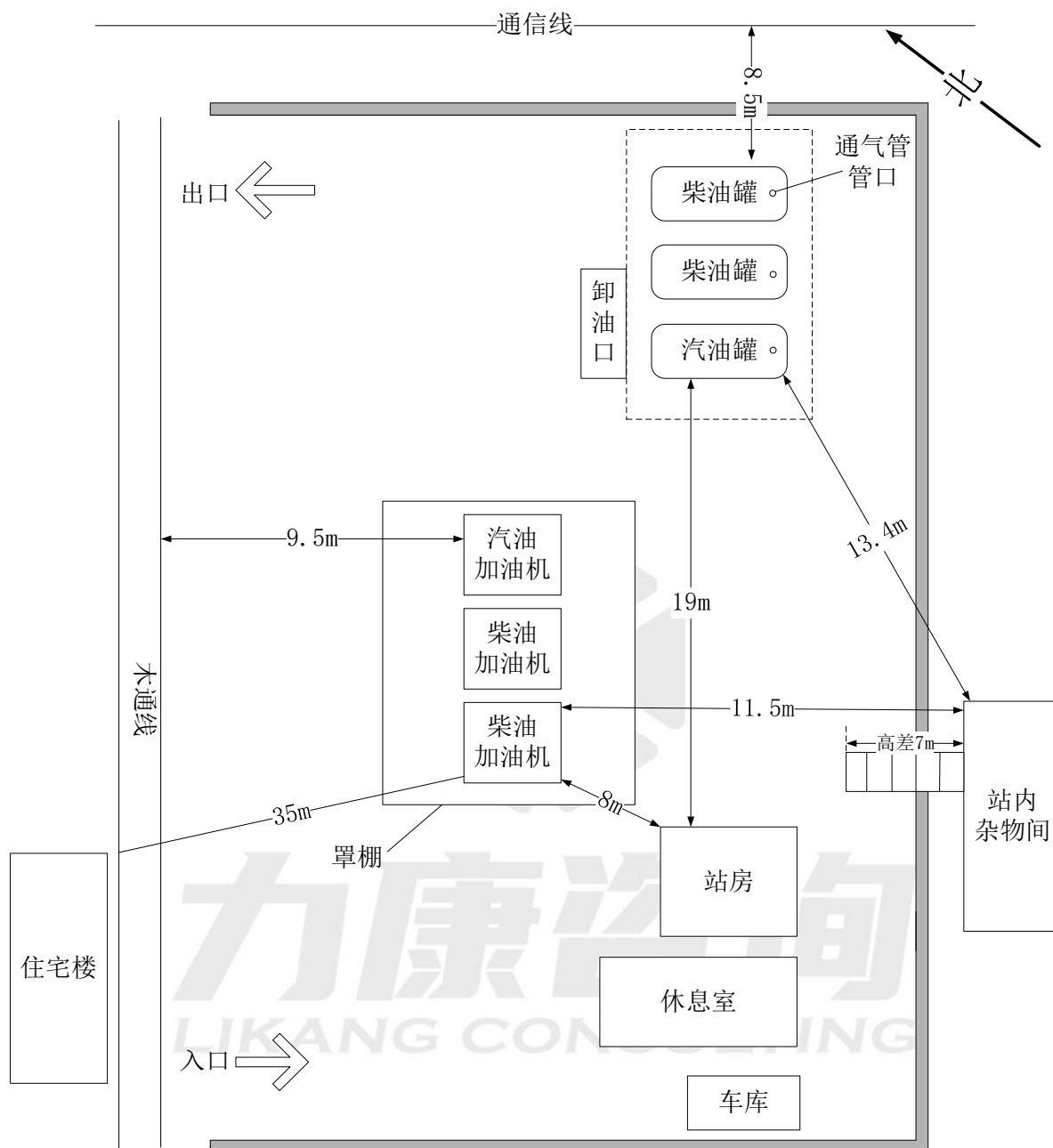
图 2.3-1 加油站周边环境和总平面布置示意图
